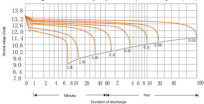
Discharge characteristics 77°F (25°C) / Caractéristiques de décharge 77°F (25°C)
