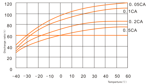
Temperature and discharge capacity / Température et capacité de décharge
